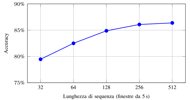
Fig. 10. Accuratezza sul validation set ufficiale al variare della lunghezza di sequenza data in ingresso alla GRU, a parità di pesi (nessun riaddestramento)
