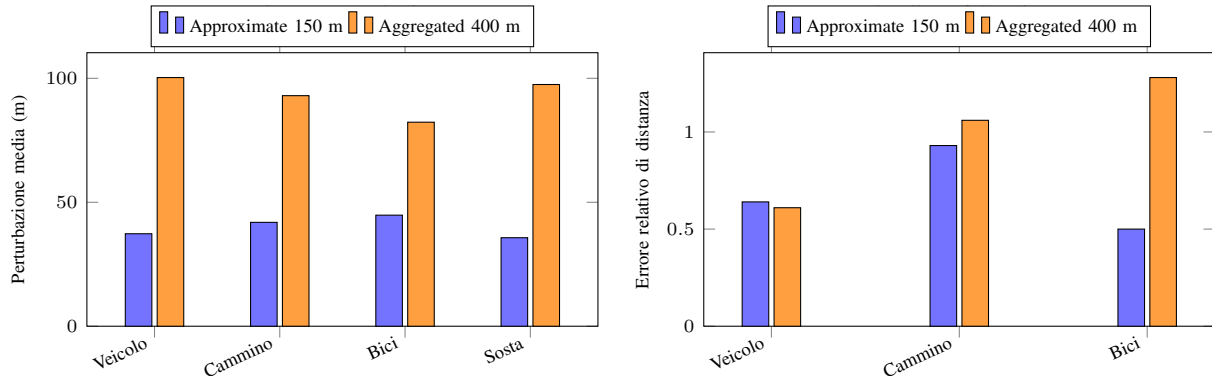
Fig. 11. Trade-off misurato tra protezione della posizione e utilità. La griglia più ampia aumenta sempre la perturbazione, mentre la distorsione della distanza dipende dalla geometria e dalla lunghezza tipica dei segmenti di ciascuna modalità.
